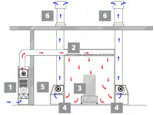
Gösterilen model: YK-SO Kapalı Kuru Filtreli Boya Kabini (Shown model)
