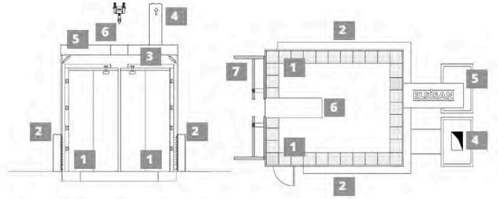
Shown model: Wash Booth with Crane Opening ( Modèle présenté )
