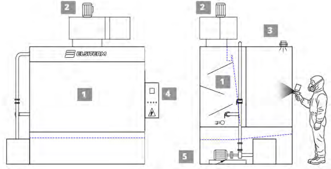
Gösterilen model: YBM Serisi Önü Açık Su Perdeli Boya Kabini (Shown model)
